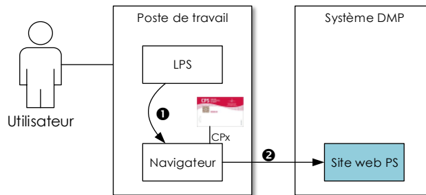
Figure 29 : architecture minimale hors DMP-compatibilité
