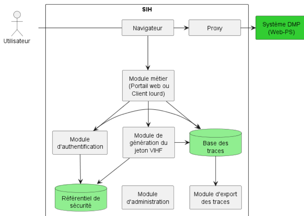
Figure 42 – Composants minimaux pour l'accès navigateur
