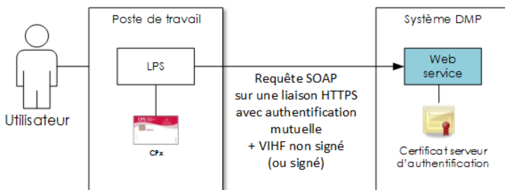
Figure 33 : authentification directe par CPx
