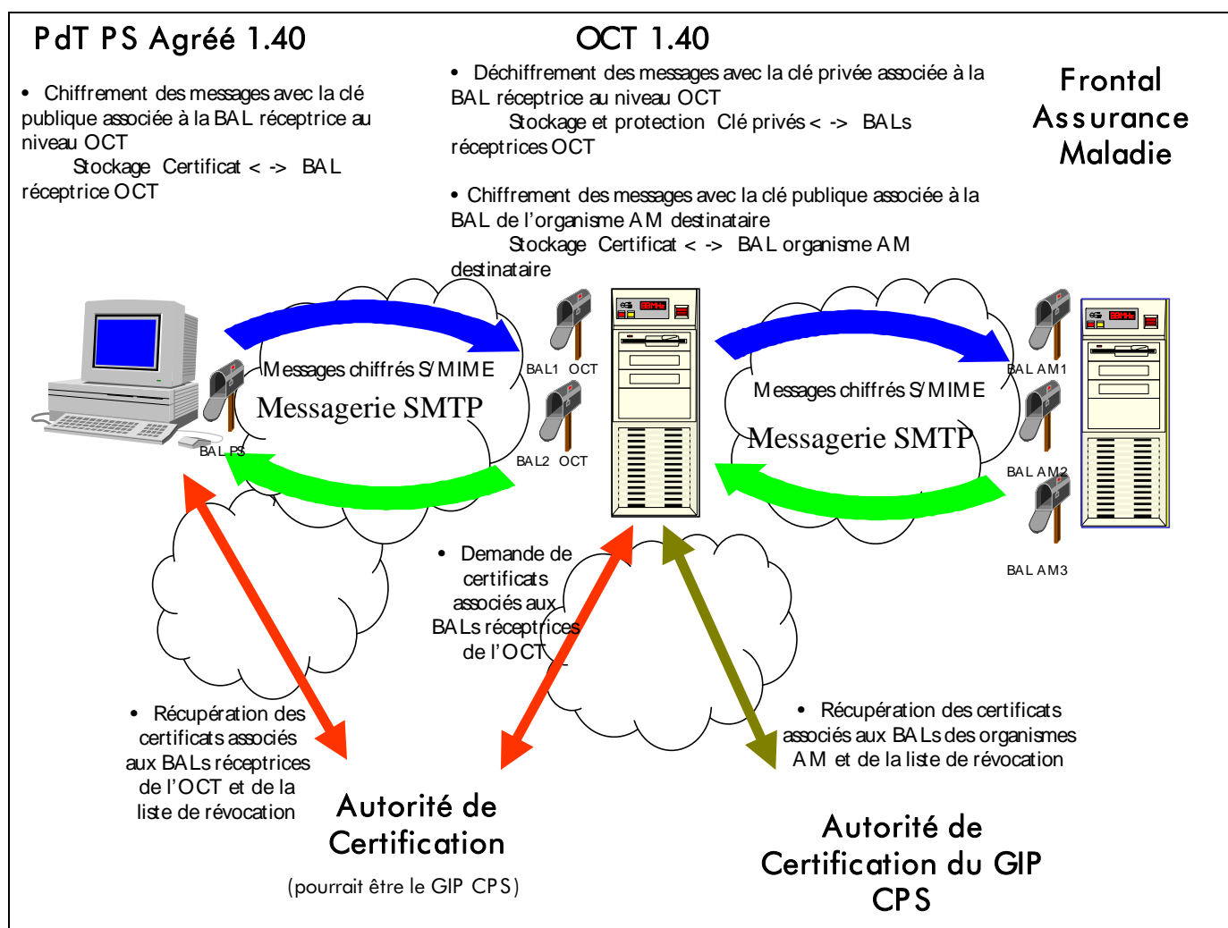
Figure 1 : Schéma du chiffrement de transport
